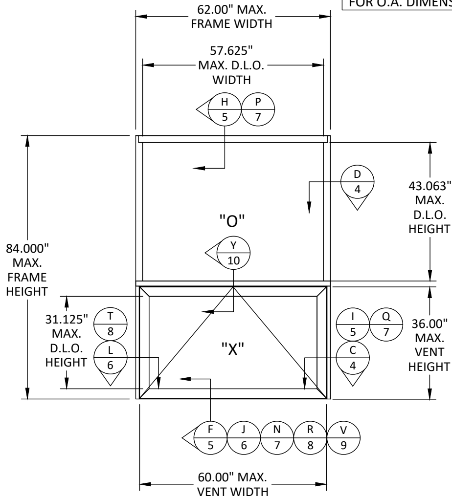
ELEVATION
