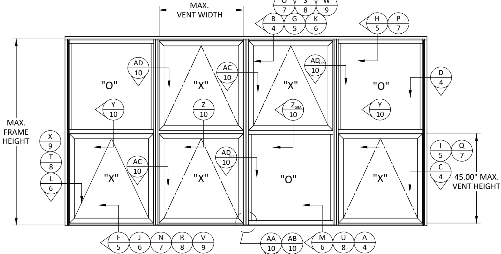
ELEVATION
